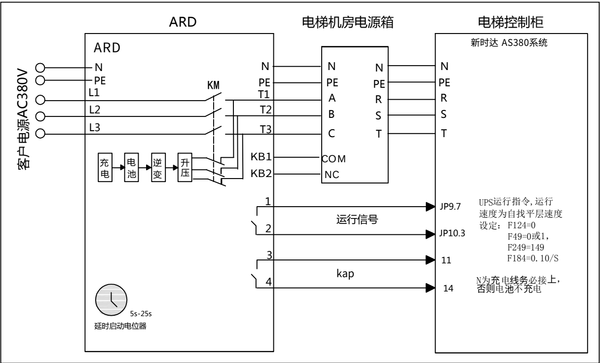
应用举例 2：新时达 AS380 一体机系统
