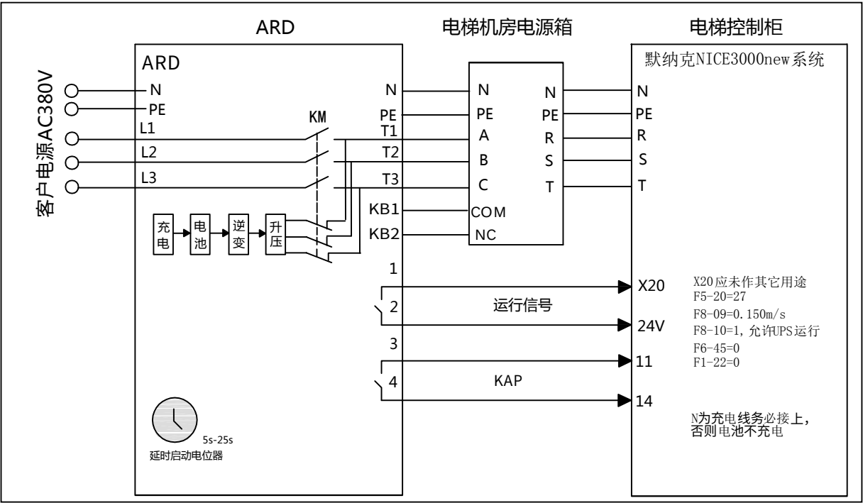
应用举例 1：默纳克 NICE3000+串行一体机系统
